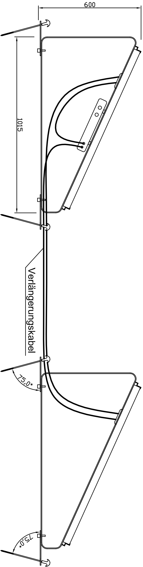
Seitenansicht
